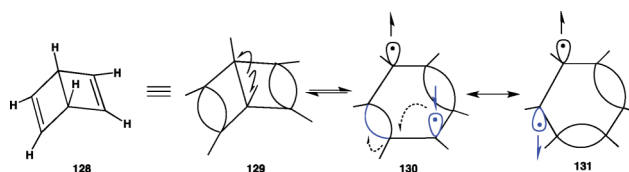
Fig. 38 Dewar benzene.
